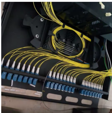
ODF -48 FO (2U)
